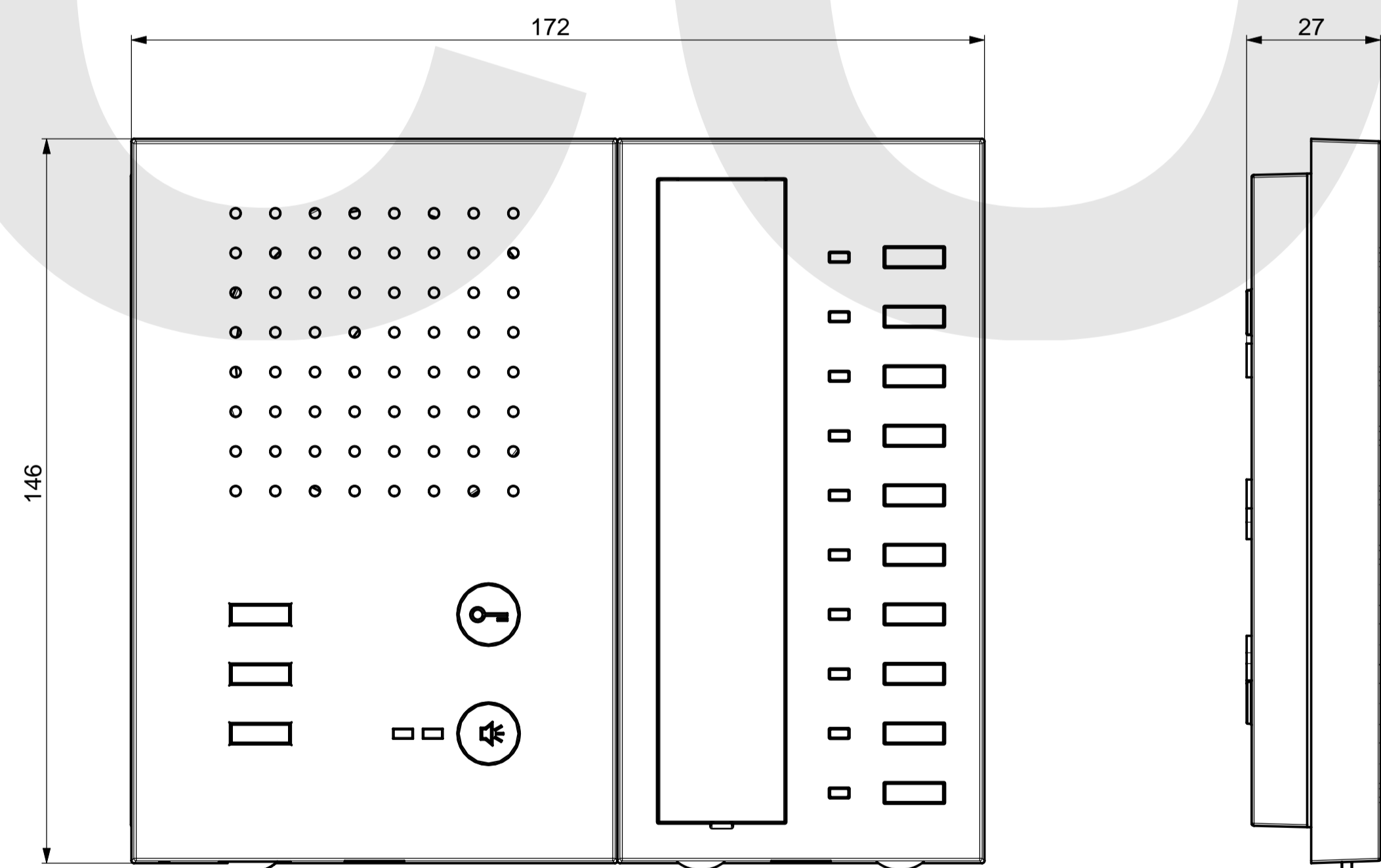
Gehäusemaß
