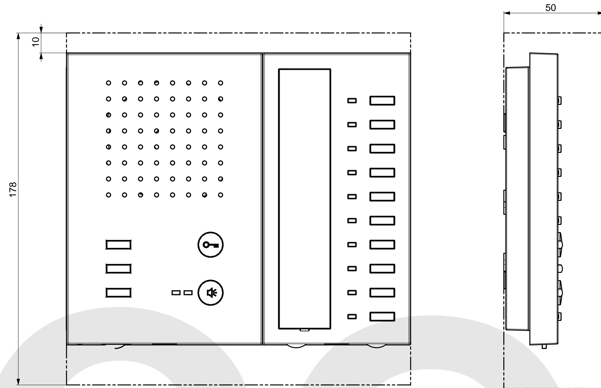
Gehäusemaß
