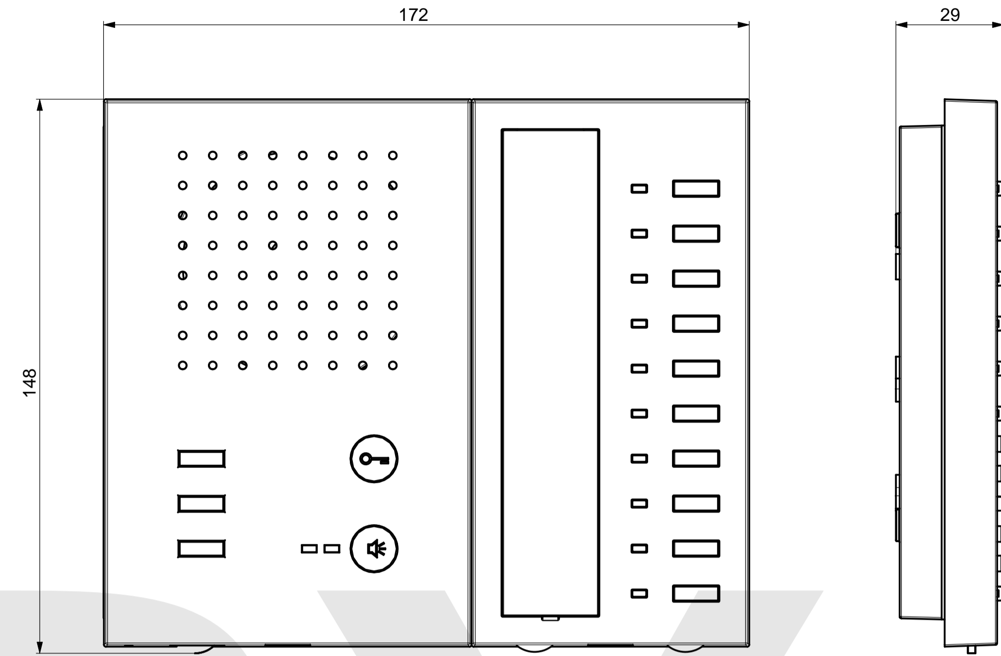
Montageansicht
