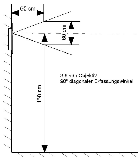
Abb. 2: Montagehöhe
