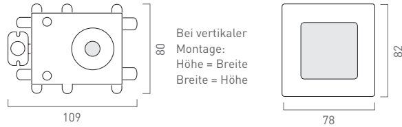
Einbau-Kamera FVK2200-0300
