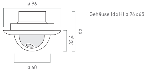
Dome-Kameramodul AMI10620-0057
