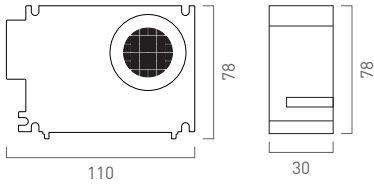
Einbau-Türlautsprecher ASI11000-0000
