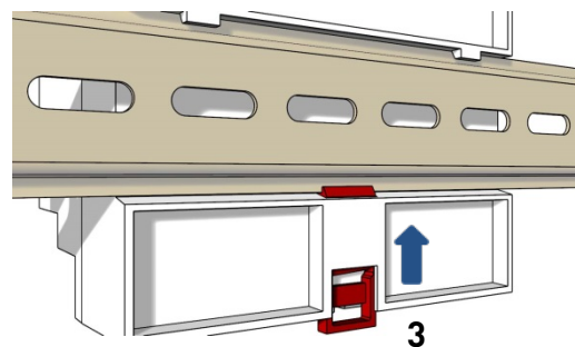
Abb. 2: Verriegelung
