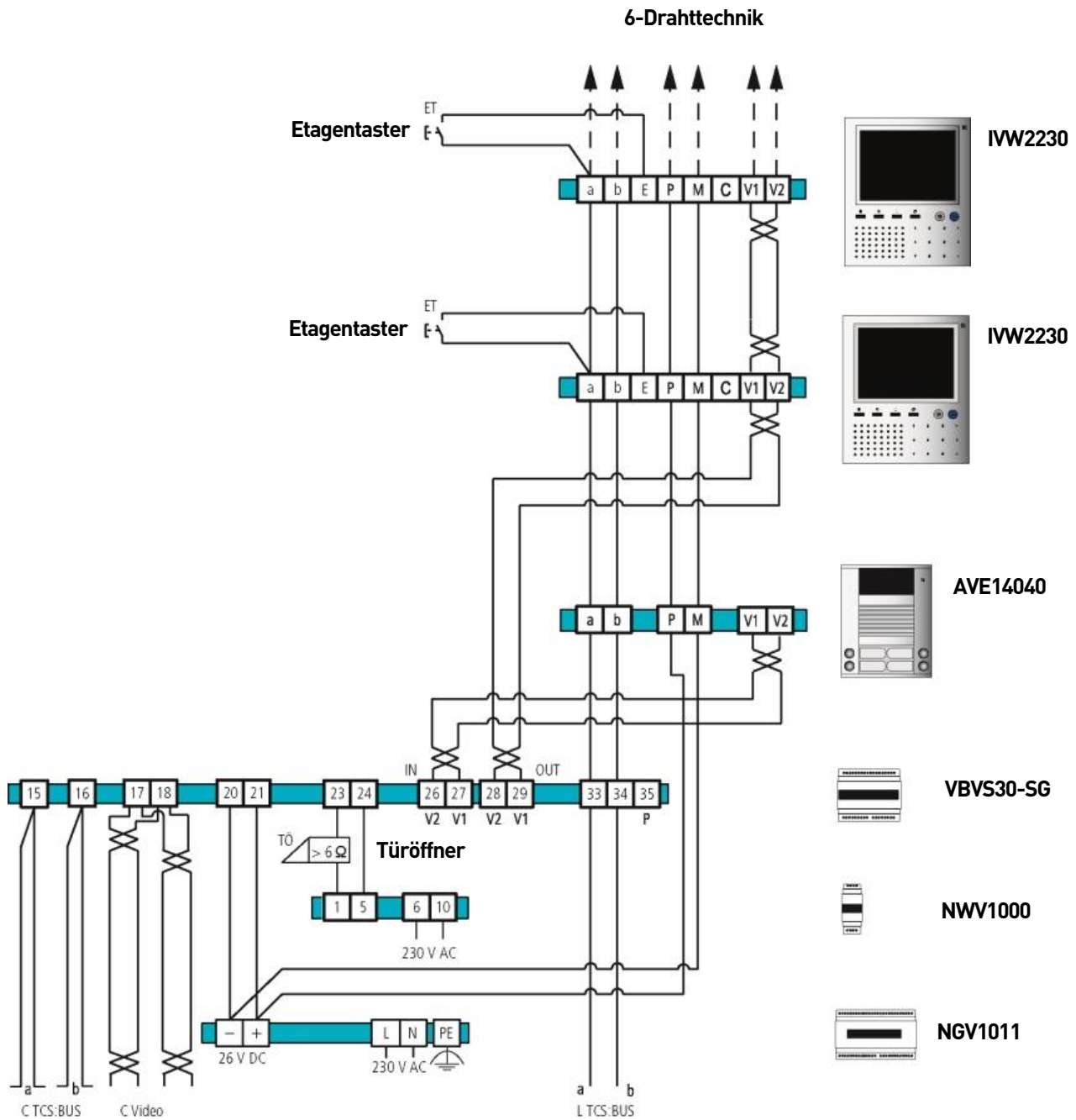
Abb. 4: Beispiel-Schaltplan
